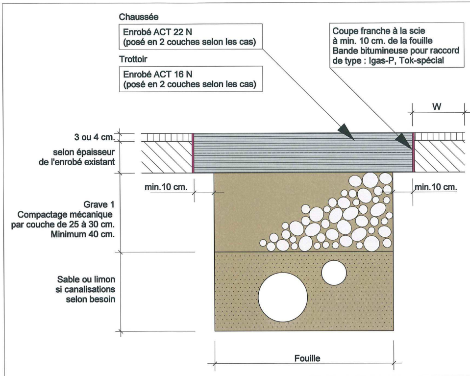
Coupe type "P": REFECTION PROVISOIRE
